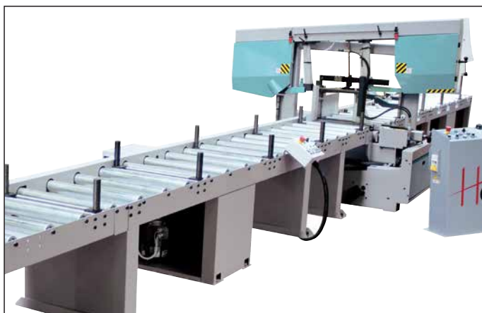
RTR rulliera motorizzata / motorized roller table - OPTIONAL
